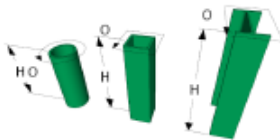
Buis- / H-Profiel O x H Minimale omtrek = 160mm Met voetplaat x 1,25 Met kap- en voetplaat x1,35
